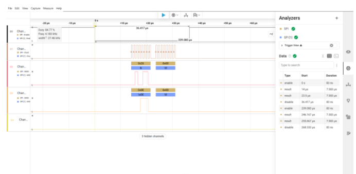
Figura 18. Modificación del registro RF_SETUP para establecer una potencia de -18dBm.
