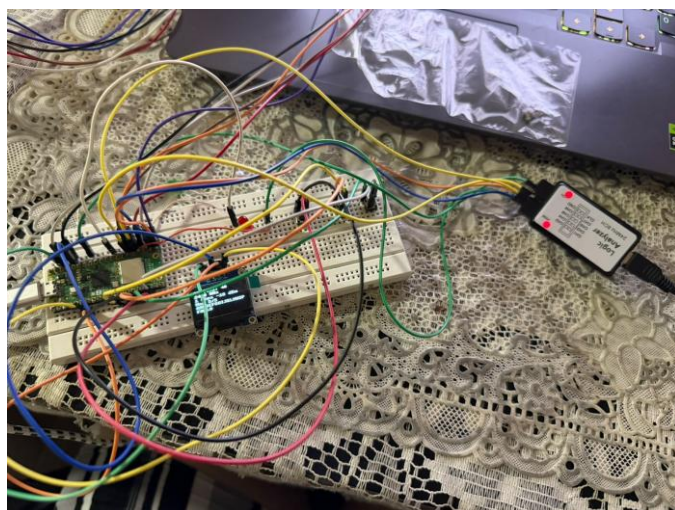
Figura 6. Conexión del analizador lógico al sistema transmisor para captura de señales SPI
