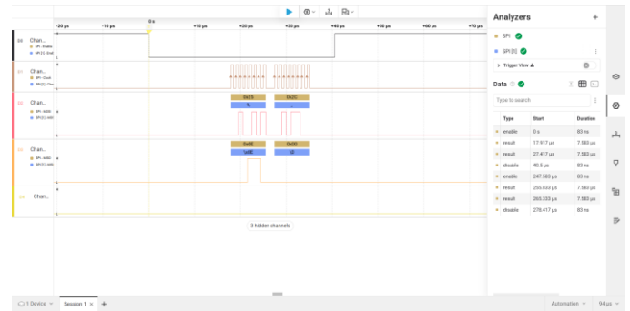
Figura 8. Operación de escritura sobre el registro RF_CH para modificar el canal de operación.
