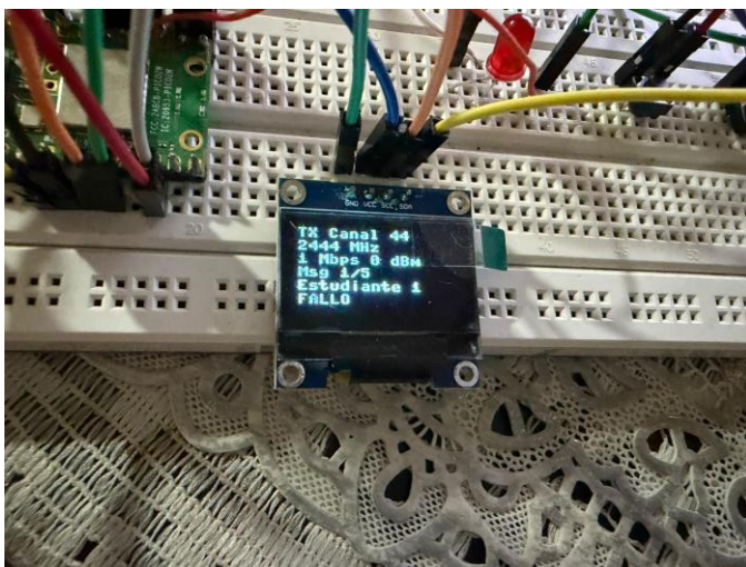
Figura 11. Indicación de fallo de transmisión en la pantalla OLED de transmisor
