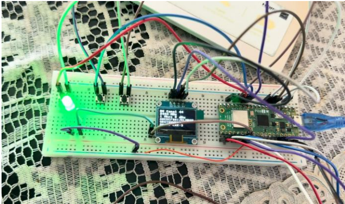
Figura 19. Recepción correcta de los mensajes en el sistema receptor.
