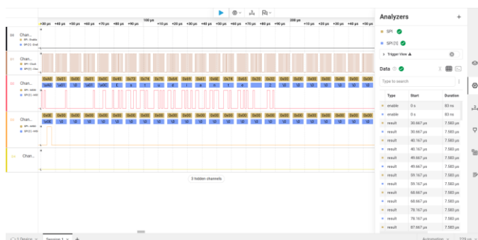
Figura 15. Transferencia del mensaje "Estudiante 2" mediante SPI.
