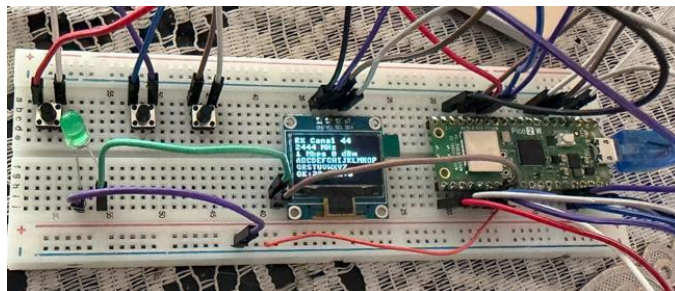
Figura 5. Montaje del sistema receptor (RX)
