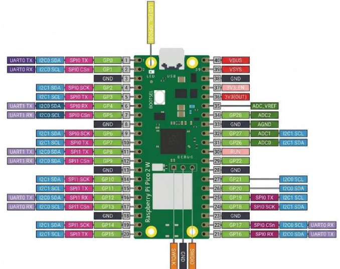
Figura 3. Ubicación de los pines en La Raspberry Pi Pico 2W.
