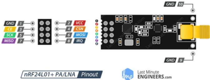
Figura 1. Identificación de los pines del módulo NRF24L01
