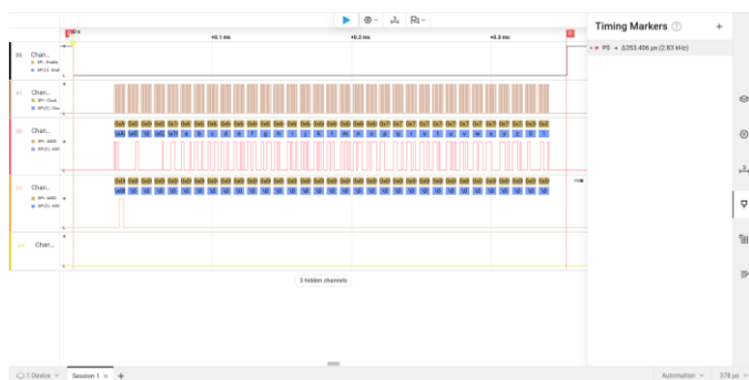
Figura 16. Primer paquete correspondiente a la transmisión de un mensaje largo.
