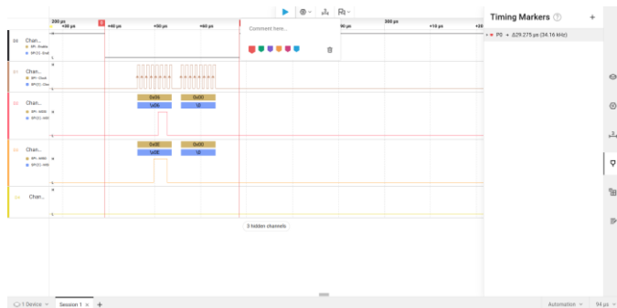
Figura 7. Captura de la operación de lectura del registro RF_SETUP mediante SPI
