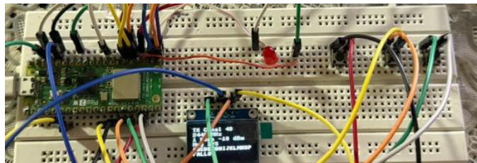
Figura 4. Montaje del sistema transmisor (TX)
